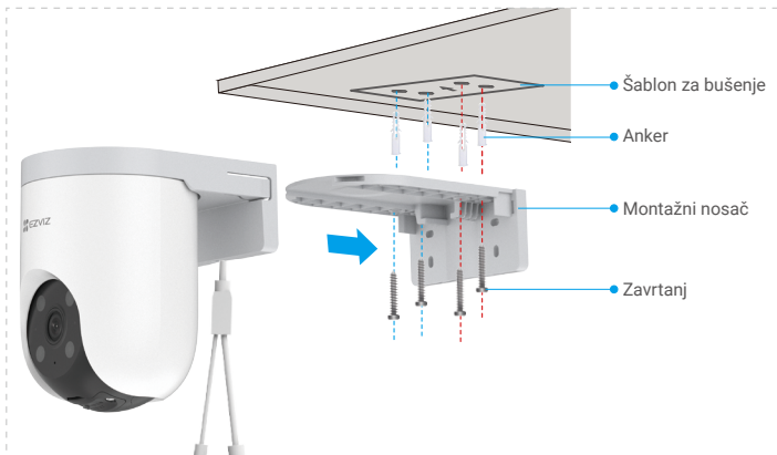
Slika 1. Montaža na plafon
